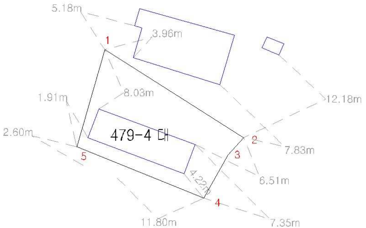
경계점 위치 설명도
